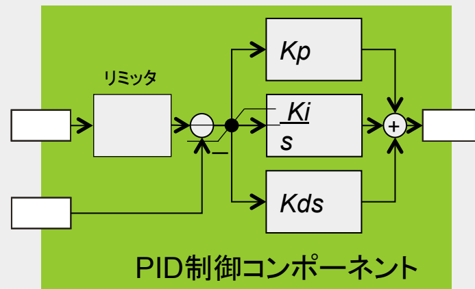
PIDコントローラの例
